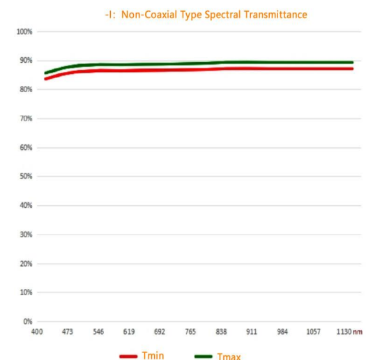
SMT11IR4W65C-I
